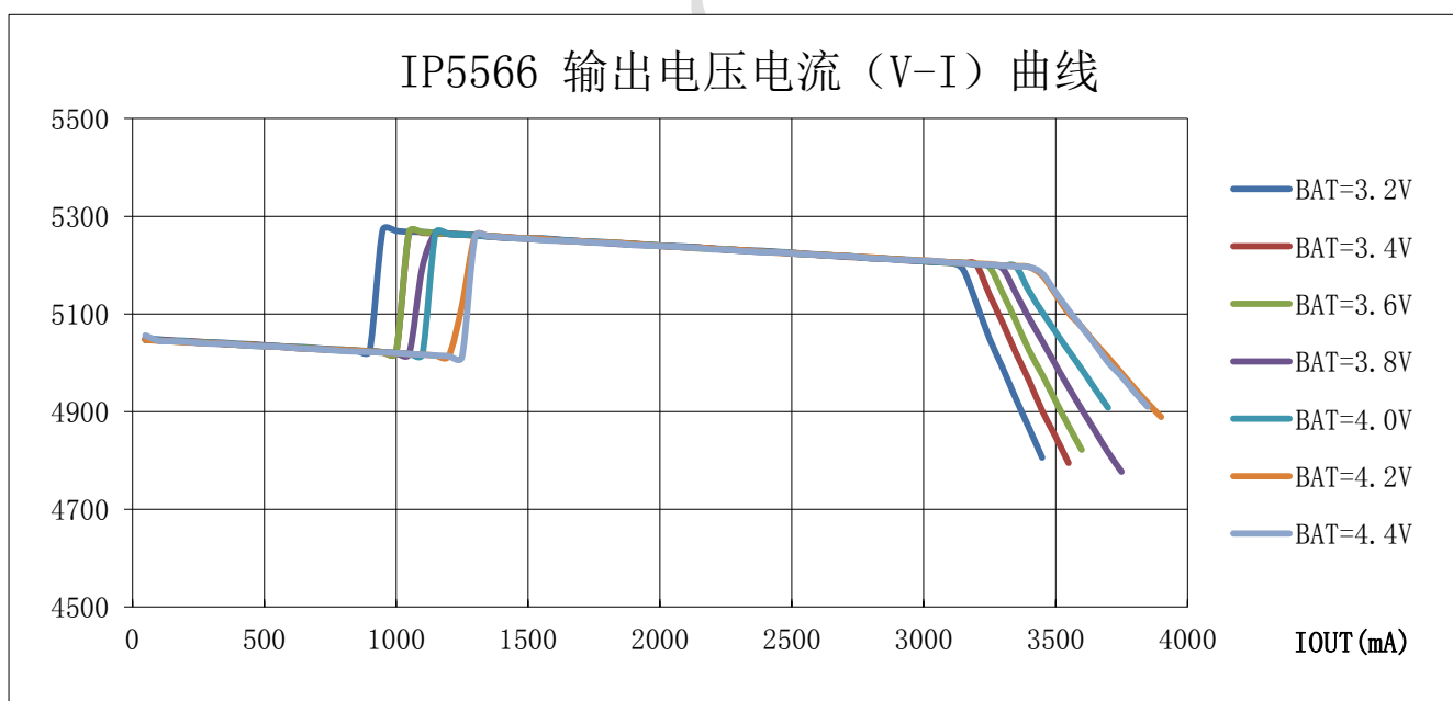
图5 IP5566 输出电压电流 (V/I) 曲线
