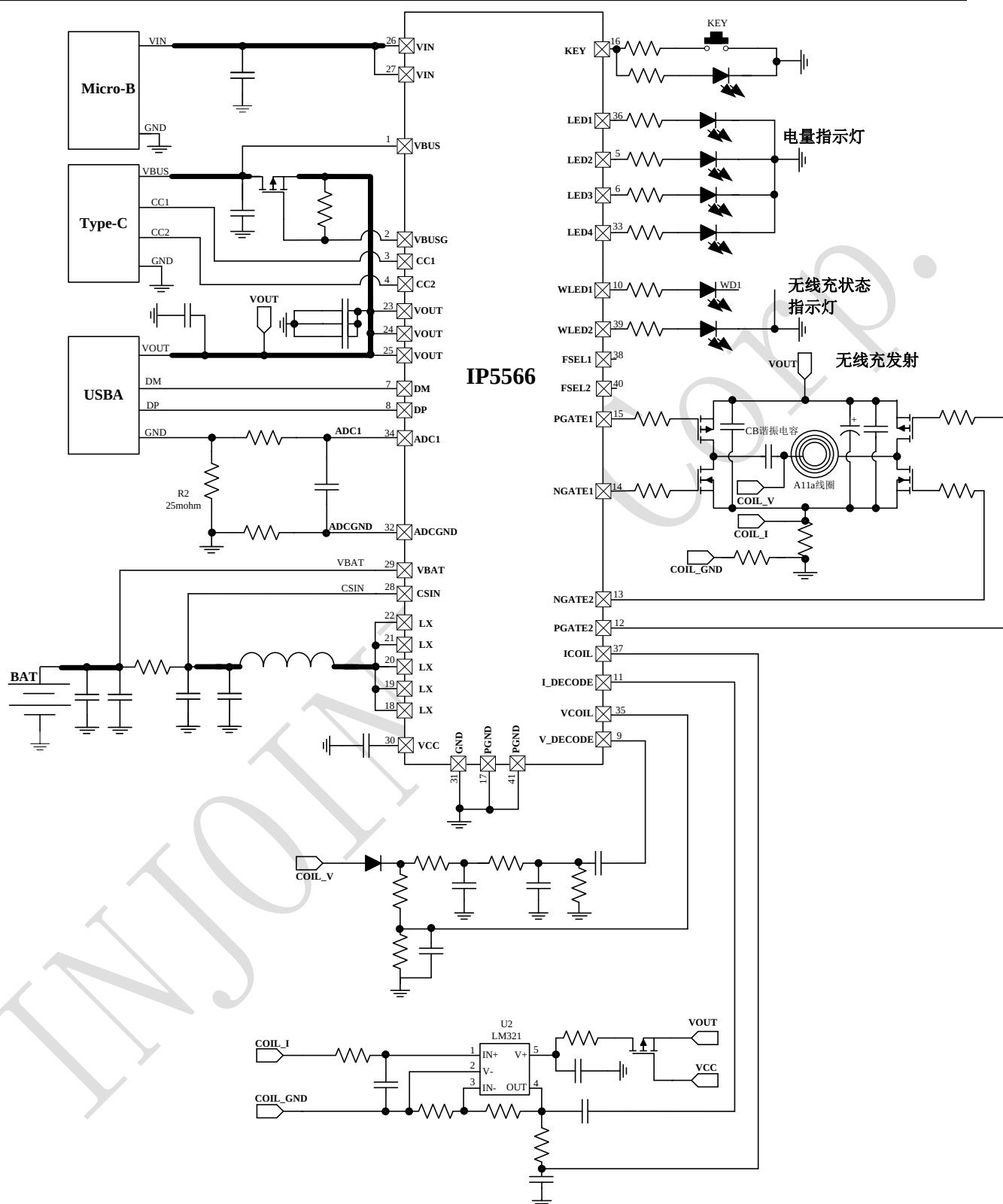
图 1 IP5566 简化应用原理图
