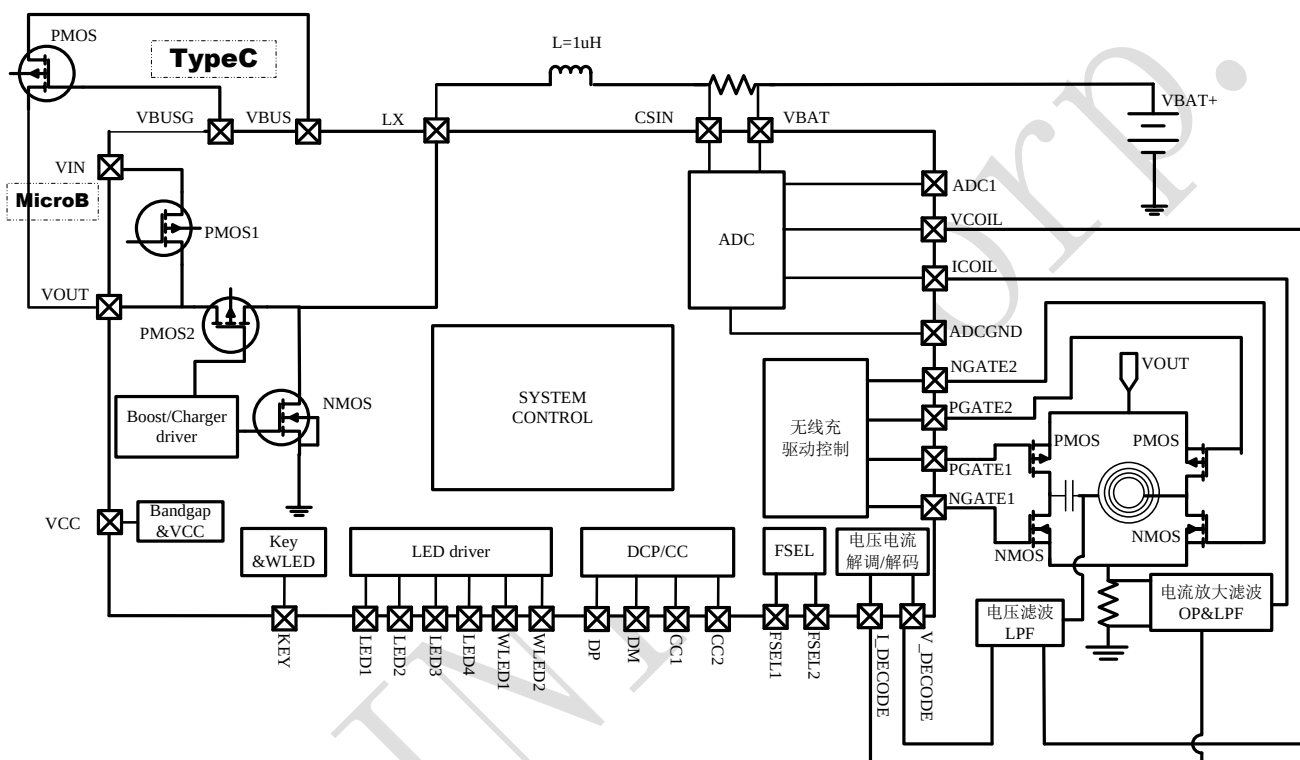
图 3 IP5566 内部系统框图
