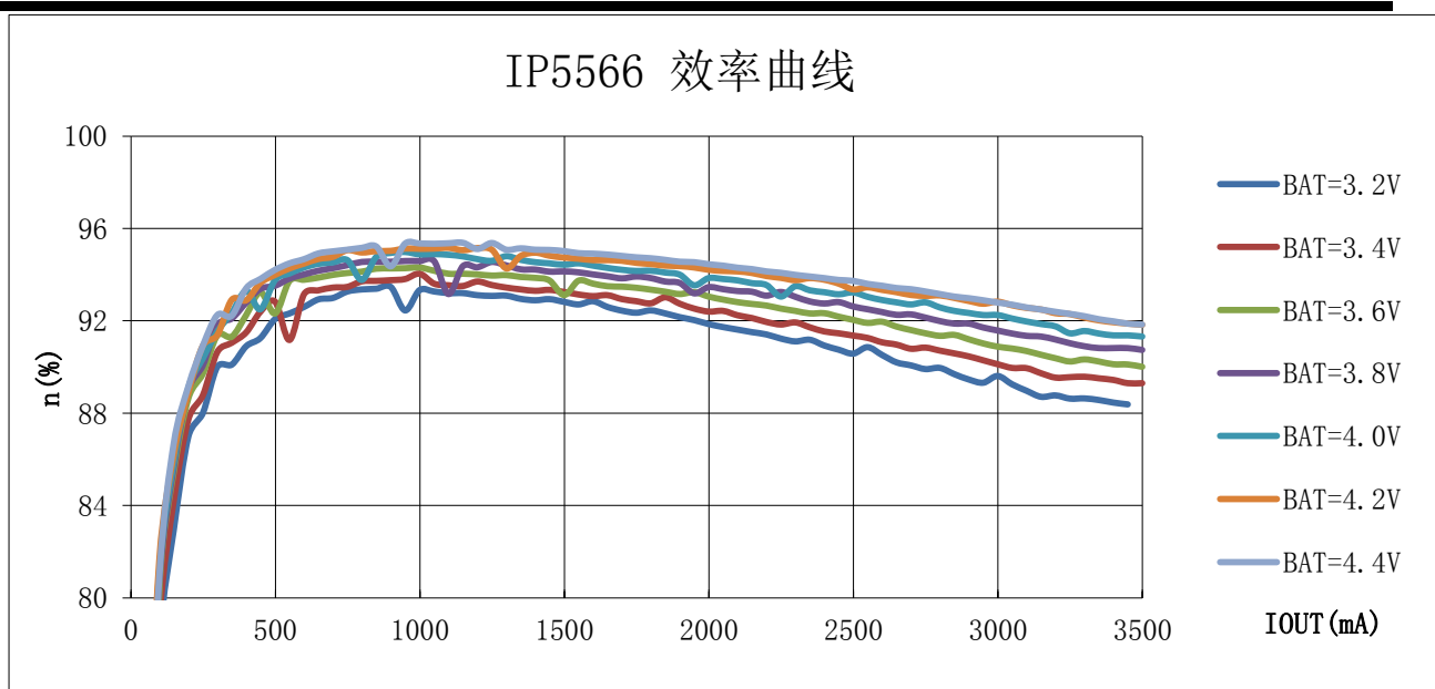
图4 IP5566 升压效率图
