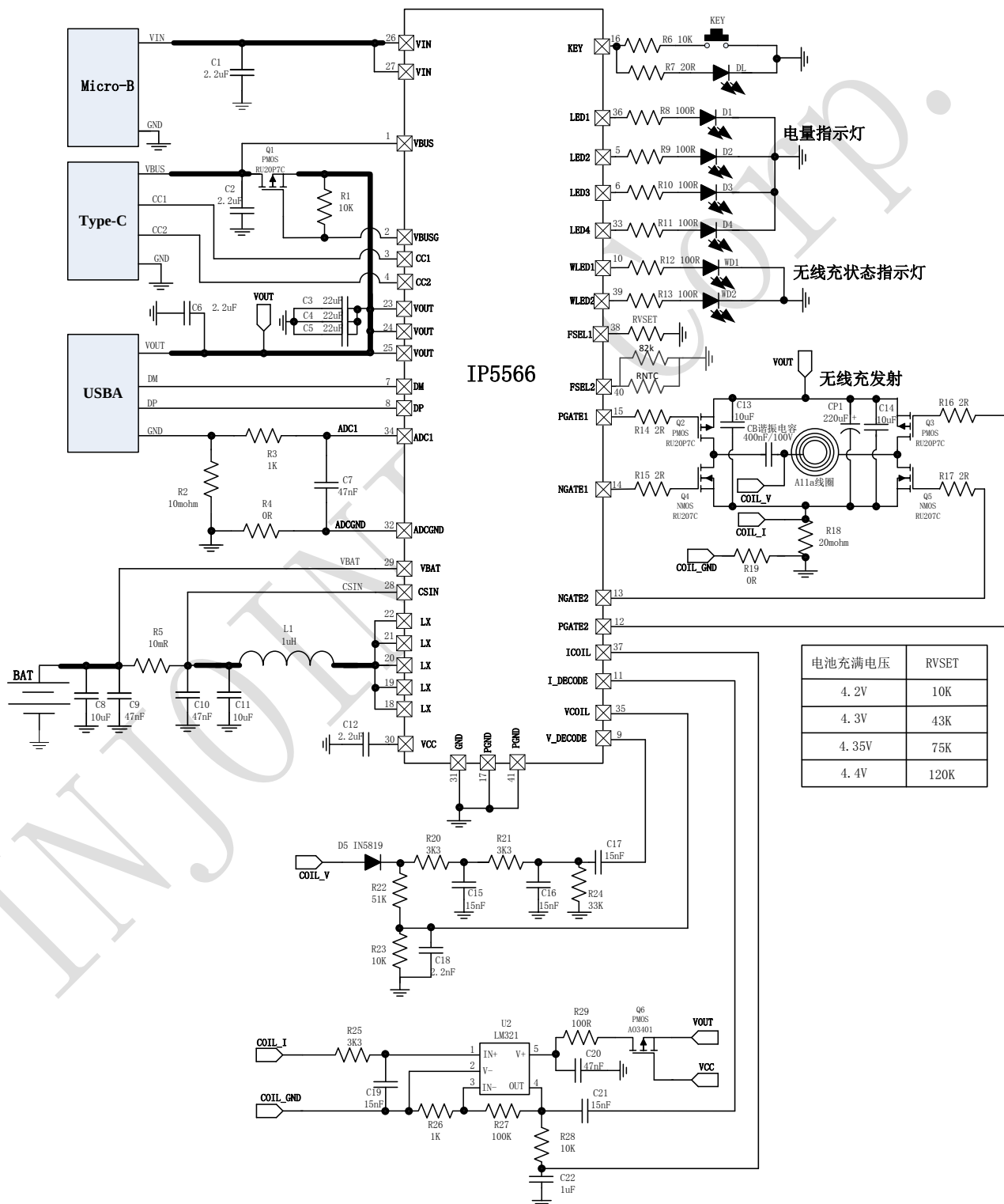
图 12 IP5566 AABC 典型应用原理图
