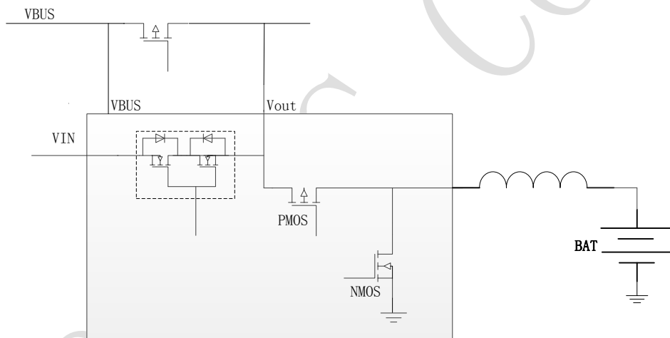
图 6 IP5566 路径管理示意图
