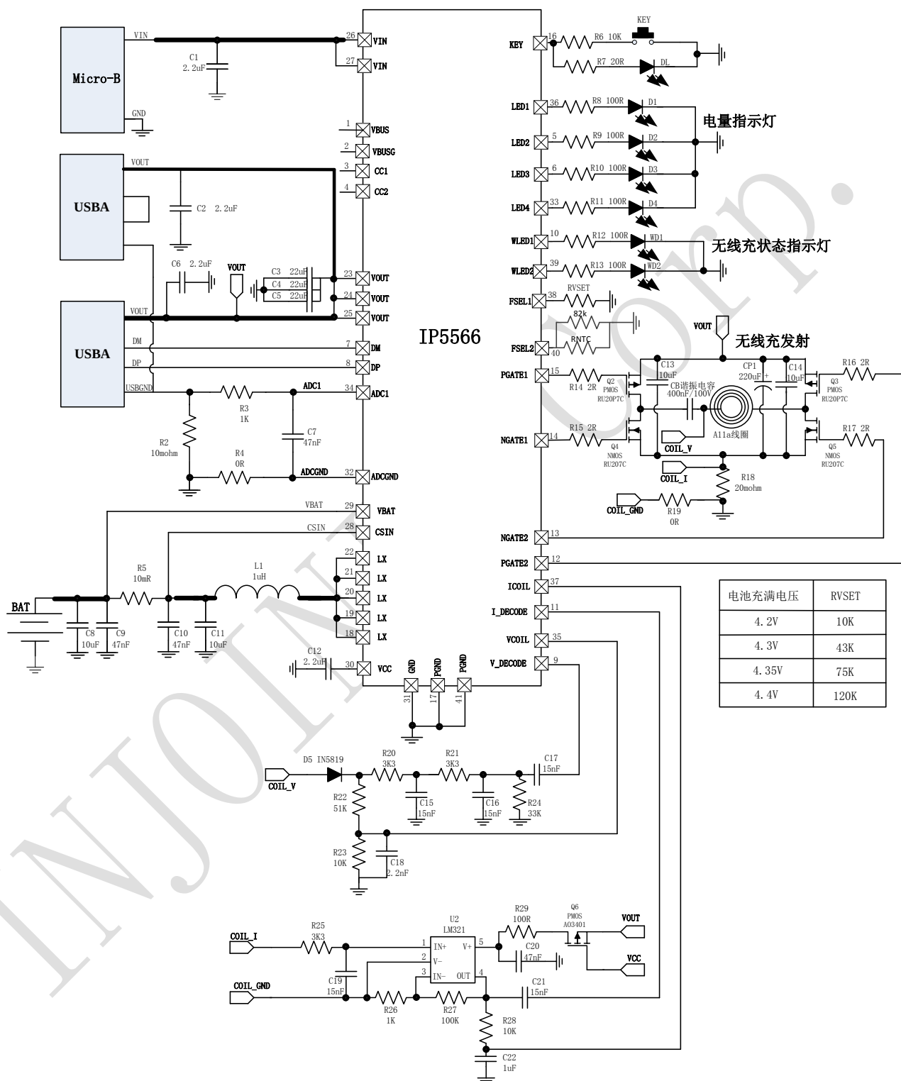
图 13 IP5566 AAB 典型应用原理图
